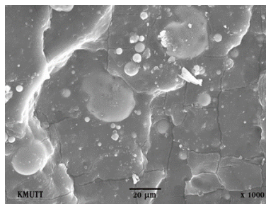
รูปที่ 2 ลักษณะพื้นผิวของอนุภาคเถ้าลอยในวัสดุผสมระหว่าง NR/SBR โดยกล้องจุลทรรศน์อิเล็กตรอนแบบส่องกราด
