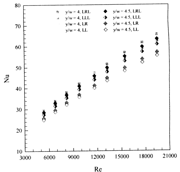
รูปที่ 1 ความสัมพันธ์ระหว่างการถ่ายเทความร้อนกับความเร็วของการไหล
